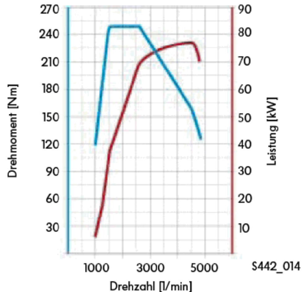
Drehmoment- und Leistungsdiagramm
